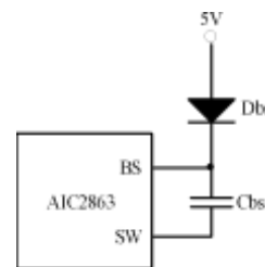
Fig. 9 Optional External Bootstrap Diode
